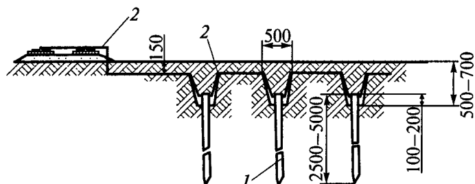
Рис. 13. Схема соединения вертикальных заземлителей: 1 — заземлитель; 2 — заземляющий проводник
