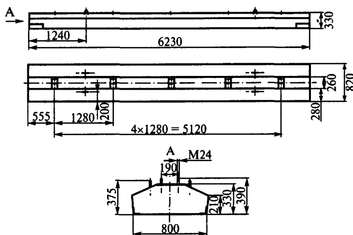
Рис. 2. Железобетонная балка типа БРП-62.8.3
