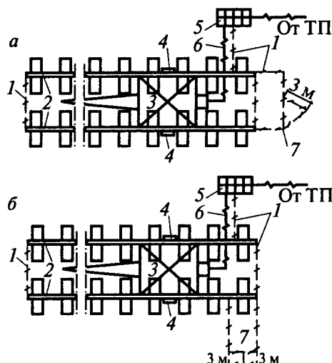
Рис. 12. Схемы заземления пути:
