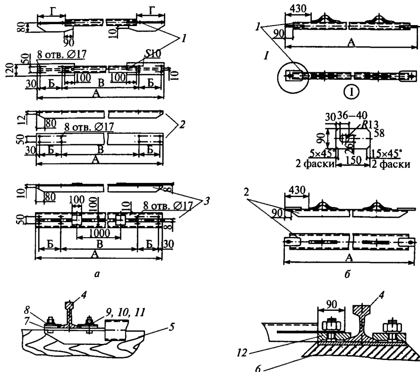
Рис. 9. Конструкции стяжек:
