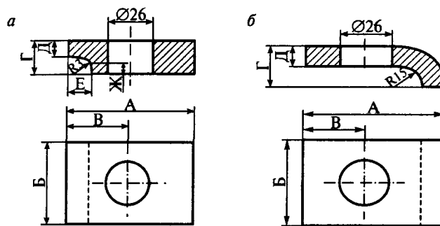
Рис. 7. Прижим:
