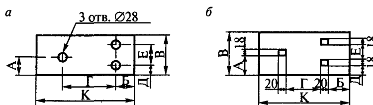
Рис. 5. Подкладки рельсов с креплением: a — с помощью шурупов; б — с помощью костылей
