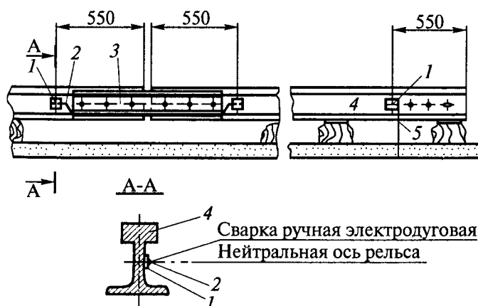
Рис. 14. Приварка заземляющих проводников и перемычек к рельсам:
