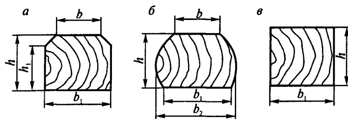
Рис. 3. Поперечное сечение деревянных полушпал: a — обрезная; б — необрезная; в — брус
