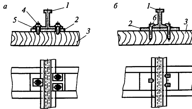
Рис. 6. Крепление рельса к полушпале:
