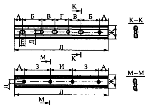
Рис. 8. Накладки двухголовые: a — шестидырные; б — четырехдырные
